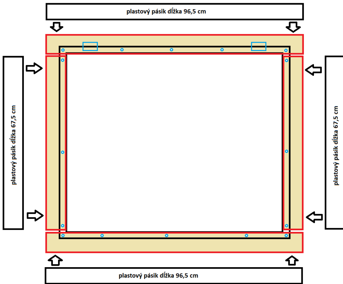
Obrázok 3 – umiestenie skrutiek
